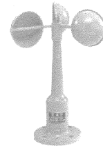
風杯型風速発信器 NS-30A
